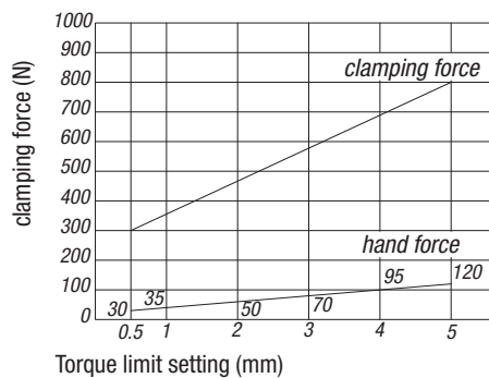
Swing Clamps 04366-...3232
