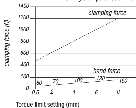
Swing Clamps 04366-...4540
